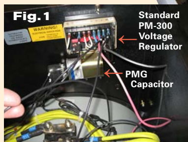
Marathon PMG Wiring
